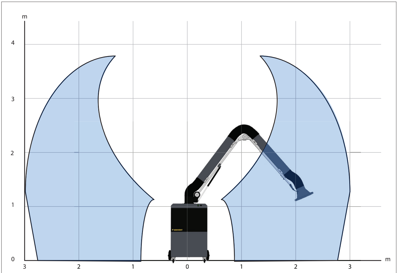
Área de trabajo para GeoGo con brazo ASA4
