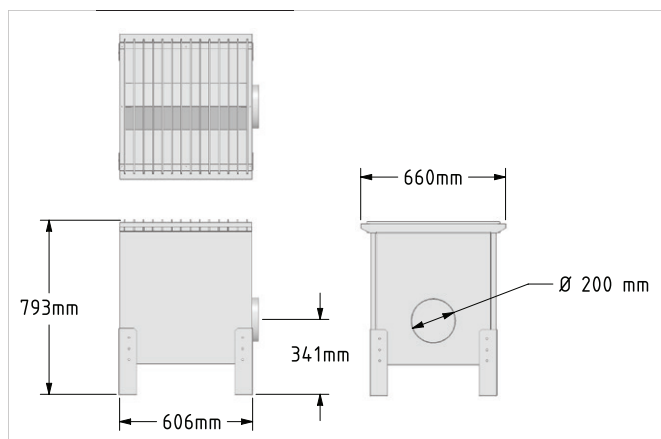
02-002 Svejsébord.
