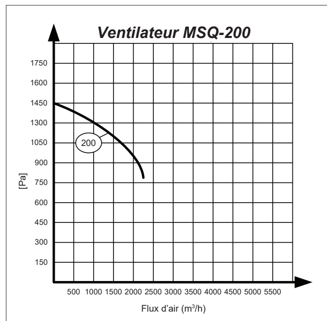
Ventilateur MSQ-200 - Extraction de point efficace
